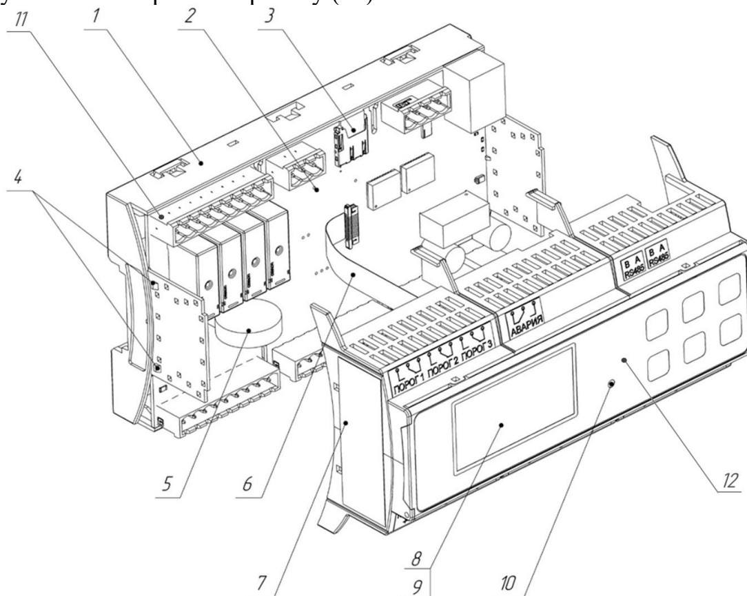
Рисунок 35 – Устройство контроллера
